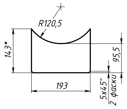
Поз.2 (Ребро)
