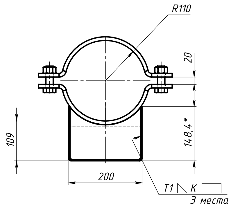
Поз.4 (Полухомут)
