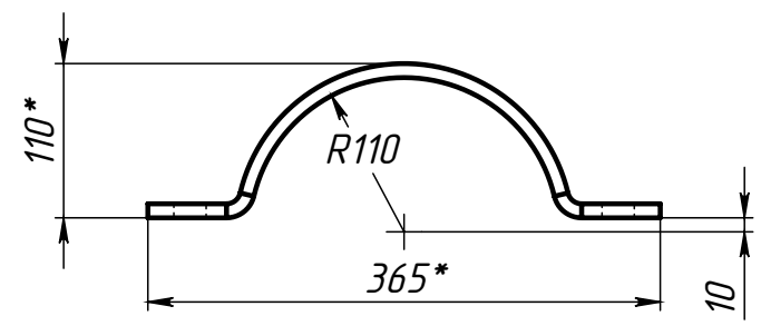
Поз.4 (Полухомут)
